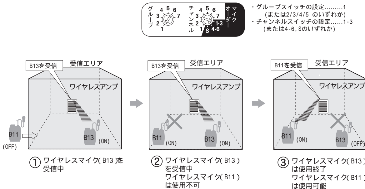
図 15 マイクオーダー運用例
